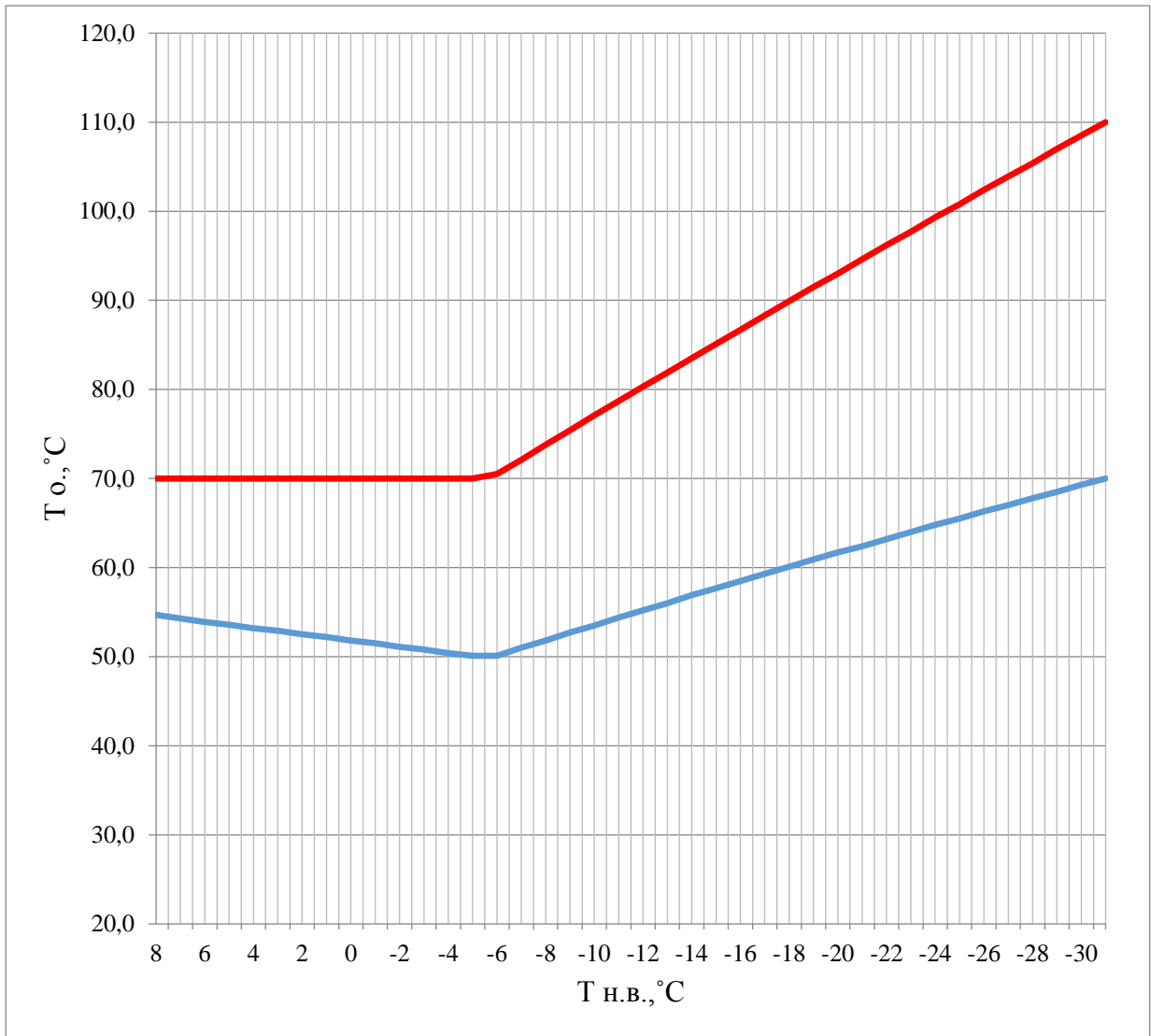
Температурный график сетевой воды для котельной ул. Никитская, 47б
